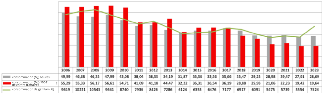
Figure 7.5.a - Consommation de gaz Pami (mégajoules/an)
